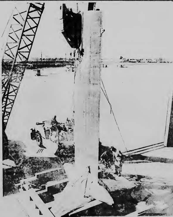
BURBANK, CALIFORNIA, --Trahadornan ta trahando riba un asina yame Sea Leg cual 'o ta capaz pa pone un cohete espacial di 300 ton den movicion (actualmente den construccion) y cu lo mester sali for di bao di awa y cu velocidad grandi.
